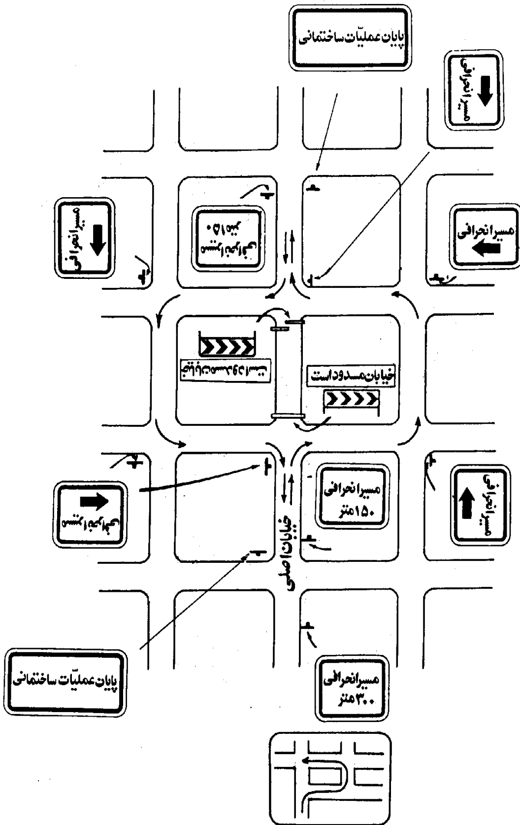
شکل ۱۲۱ . به کارگیری تابلوهای انحراف مسیر در خیابان ، در حال عملیات ساختمانی
