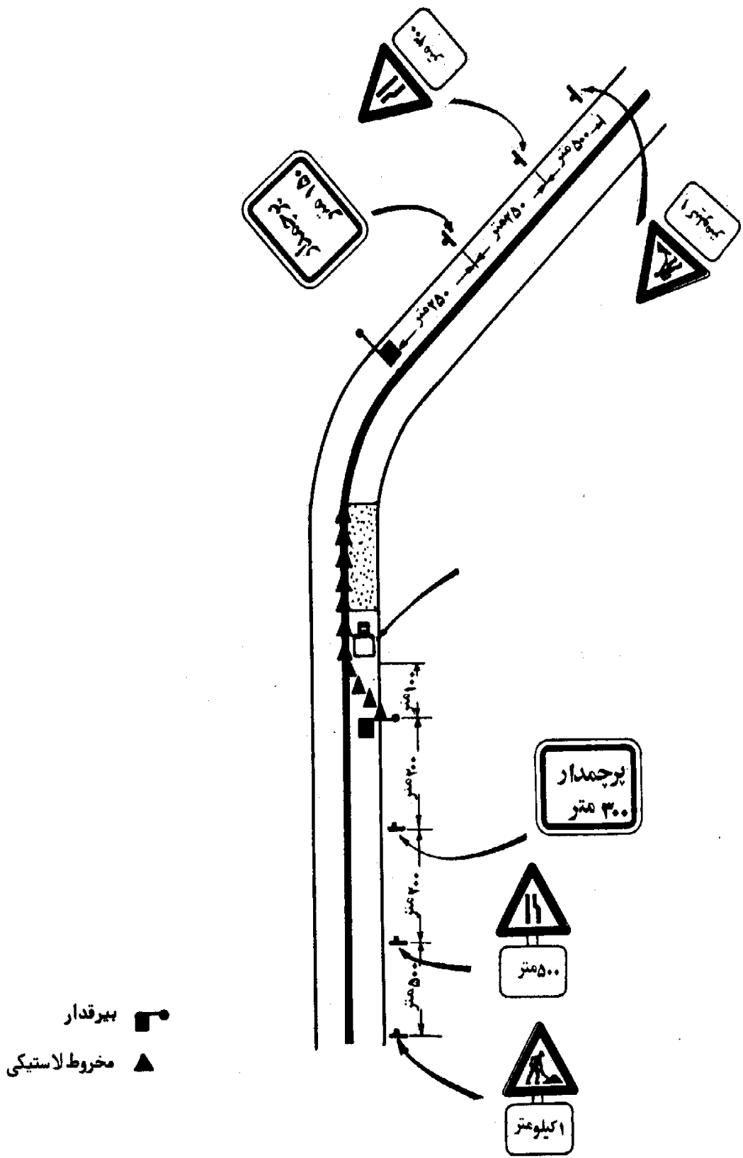
شکل ۱۲۳. علامت‌گذاری جاده دوطرفه در دست تعمیر
