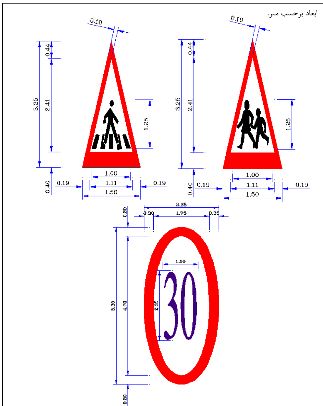
شکل ۳- نمایی از نمادهای مورد استفاده در فرایند آرامسازی ترافیک (طبق بند ۲-۹).
