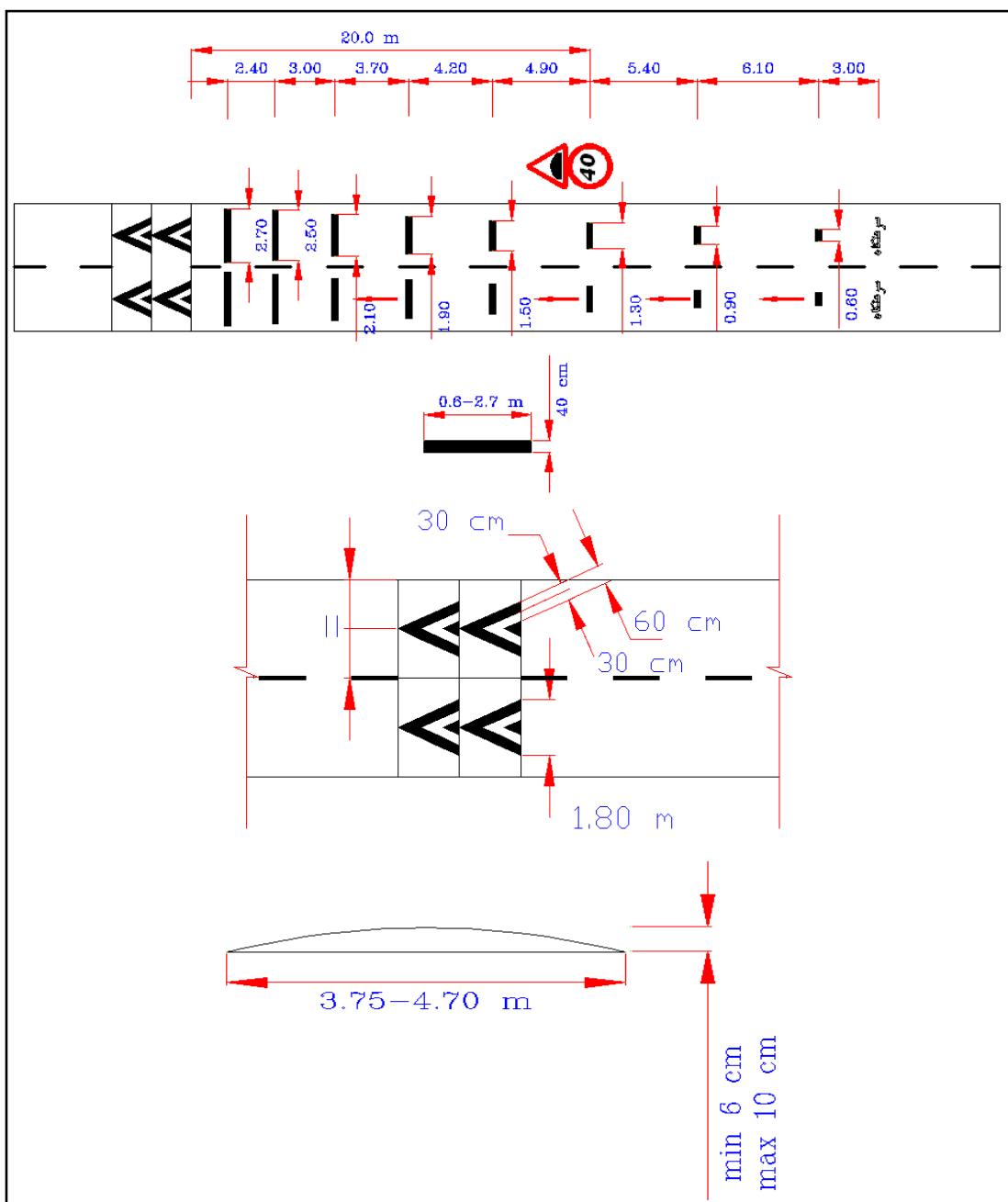
شکل ۳۷- نمایی از مشخصات اجرایی سرعت‌کاه‌های قوسی (طبق بندهای ۲-۲، ۲-۳، ۲-۴)
